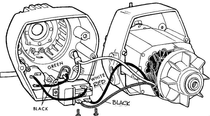
MOTOR WIRING
